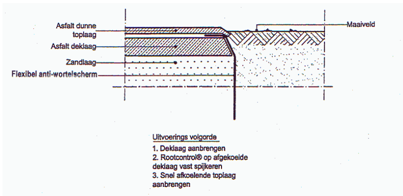
Figuur 9-19-7 (detail 1b): hoogte niveau flexibel anti-wortelscherm toepassing bij bitumineuze verharding
