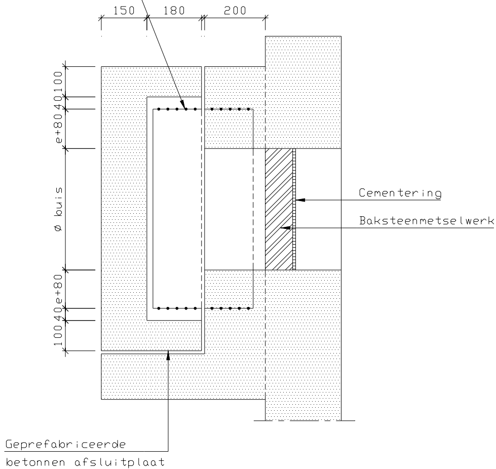
Figuur 9-17-1: detailtekening (alle maten in mm)
