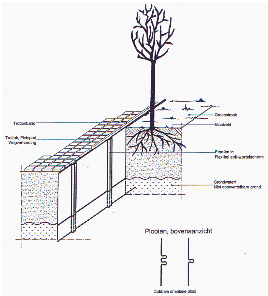
Figuur 9-19-12 (detail 3): plooiën in flexibel anti-wortelscherm
