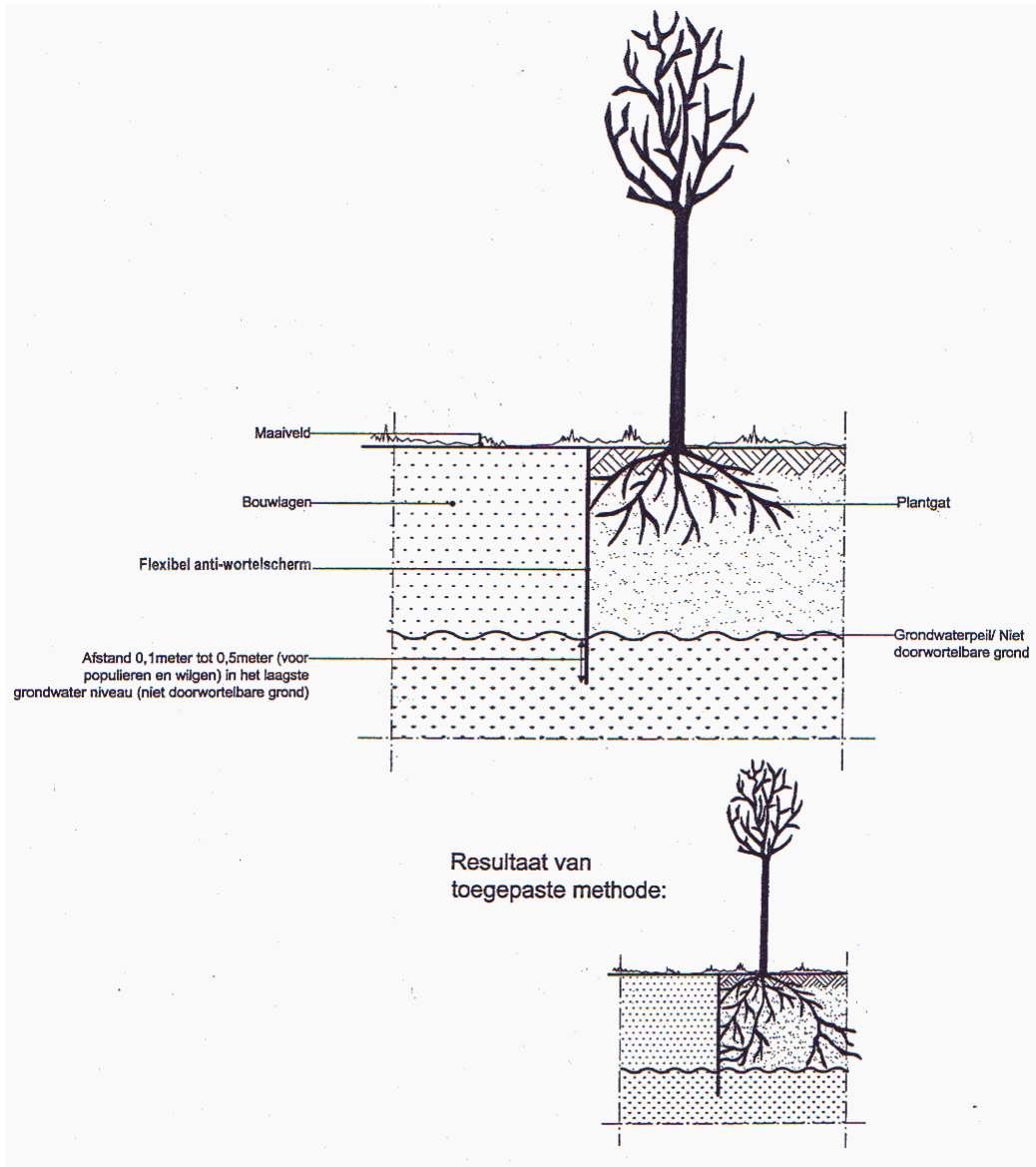
Figuur 9-19-10 (detail 2a): diepte niveau flexibel anti-wortelscherm: barriërvorming door diepe toepassing
