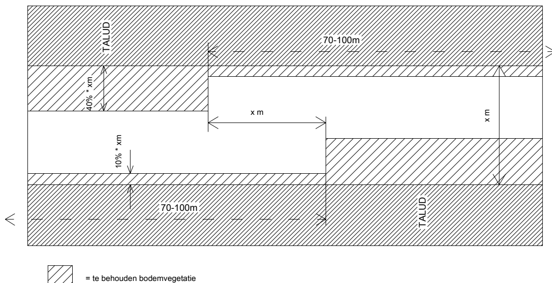
Figuur 13-1-1: schematische voorstelling van bodemmaaiing in blokken
